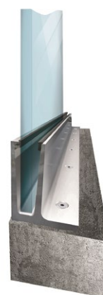
Balustrada TRAPANI Profil BAL F – montaż do podłogi z mocowaniem bocznym
