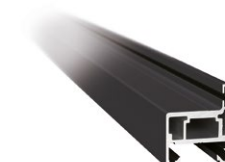
Profil ościeżnicowy typu „H”
