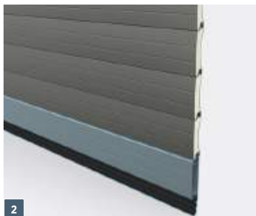
2 Profil dolny – aluminiowy profil wzmacniający o wysokości 115 mm standardowo malowany w kolorze kurtyny bramy.
