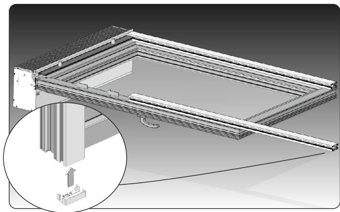
15. Nasunąć prowadnicę na przykręcone wcześniej do ramy okiennej nypie. Nałożyć i przykręcić na prowadnicę zatyczki dolne.
